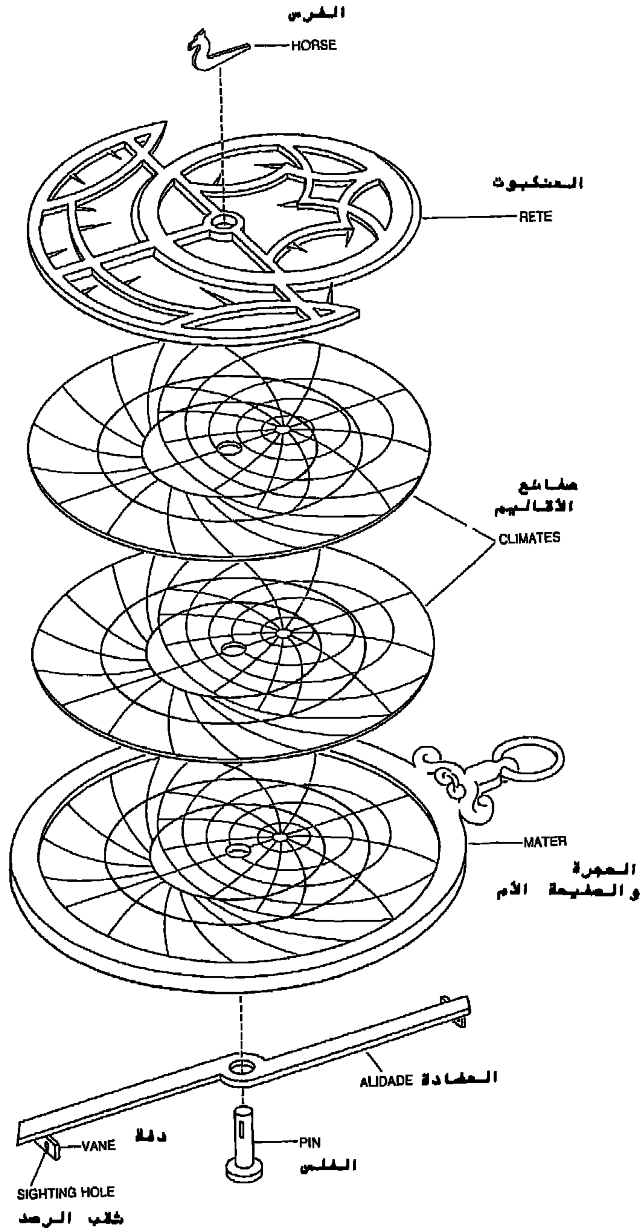
شكل (١٤,٣): أجزاء الأسطرلاب.
