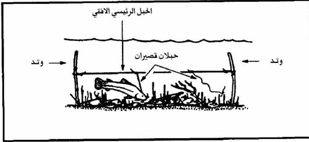
شكل 8- 18 الصيد بالوتاد
