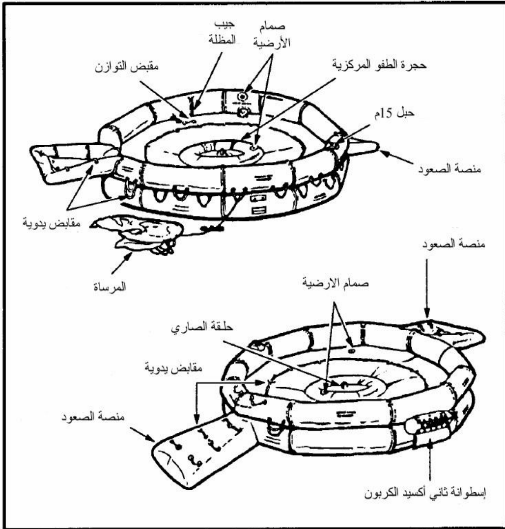
شكل 16-15 قارب النجاة لـ 20 شخص
